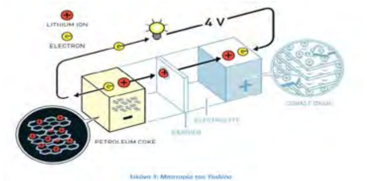
Εικόνα 3: Μπαταρία του Yoshino
