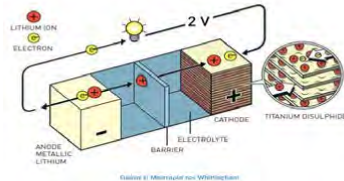
Εικόνα 1: Μπαταρία του Whittingham
