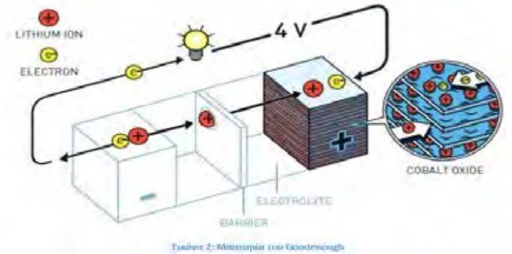
Εικόνα 2: Μπαταρία του Goodenough
