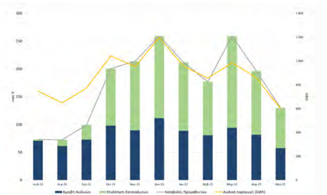
Διάγραμμα 3 : Οι πράσινες μπάρες αντιστοιχούν στις επιδοτήσεις που έχουν προσφέρει τα υφιστάμενα αιολικά πάρκα στους καταναλωτές
