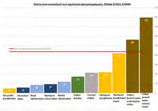
Διάγραμμα 1: Τα νέα αιολικά και τα νέα μεγάλα φωτοβολταϊκά είναι η πιο φθηνή μορφή ηλεκτροπαραγωγής
