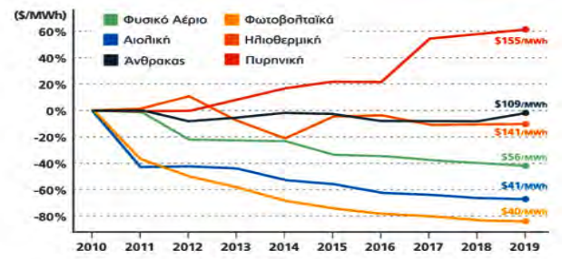
Σημ.: Το κόστος ενέργειας αφορά το σταθμισμένο κόστος παραγωγής ενέργειας (LCOE). Το φυσικό αέριο αφορά μονάδες συνδυασμένου κύκλου. Τα φωτοβολταϊκά αφορούν κρυσταλλικά πάνελ μεγάλης ισχύος.
